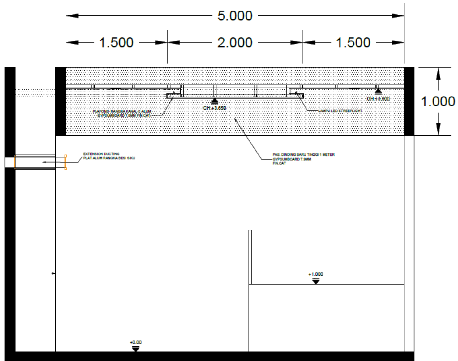
POTONGAN A-A
