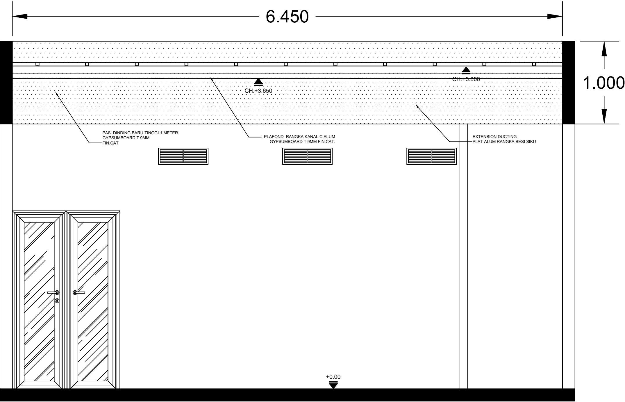
POTONGAN B-B
