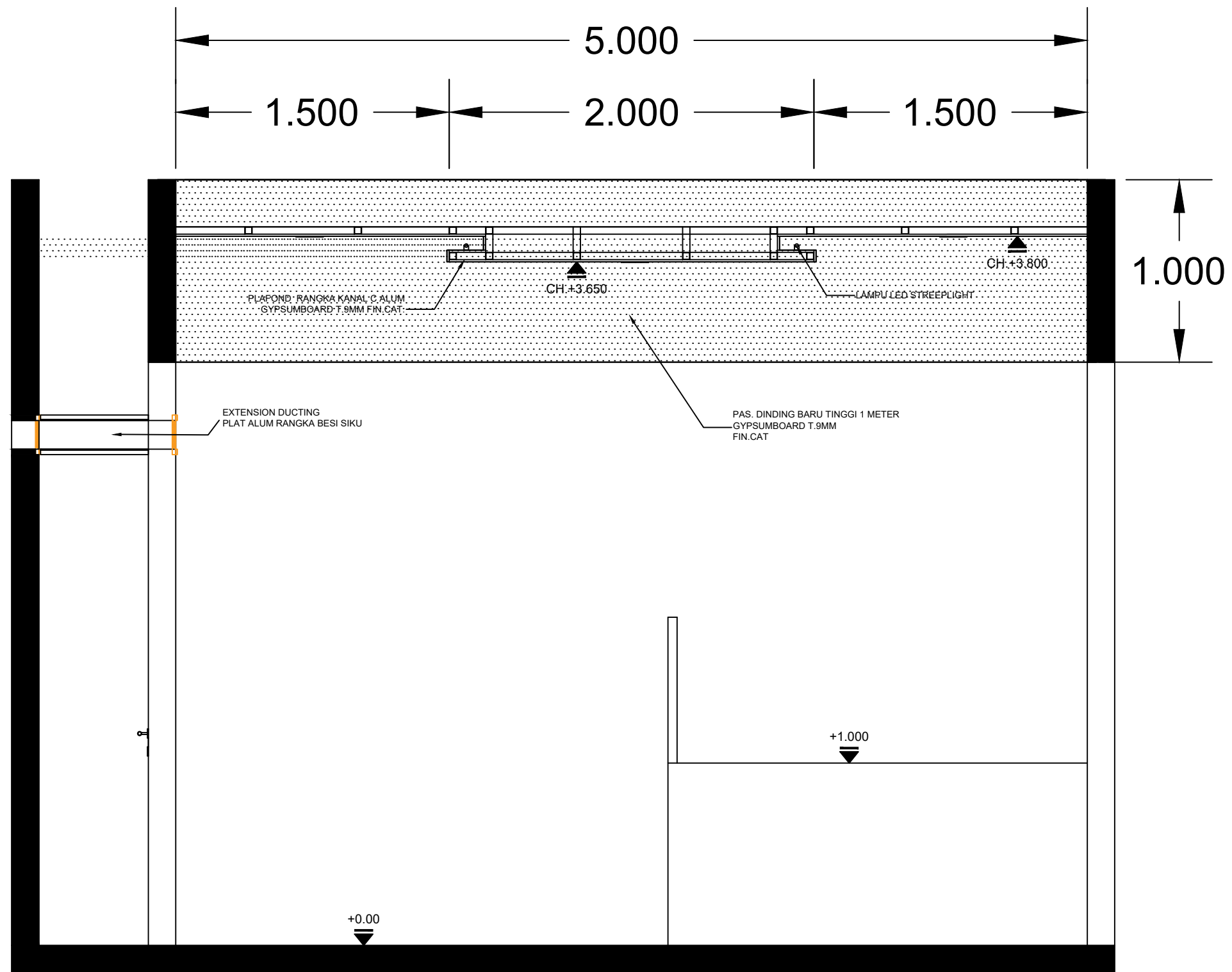
POTONGAN A-A
